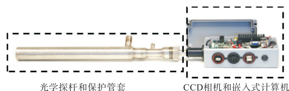
图 2 火焰图像采集系统
