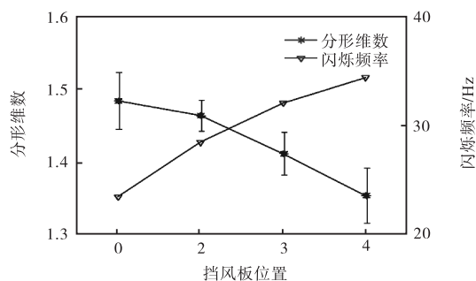
图 6 挡风板位置与热混合层分形维数、火焰闪频关系
